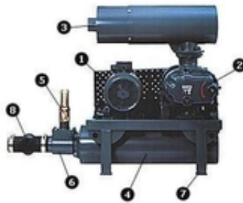
воздуходувка 2AF
